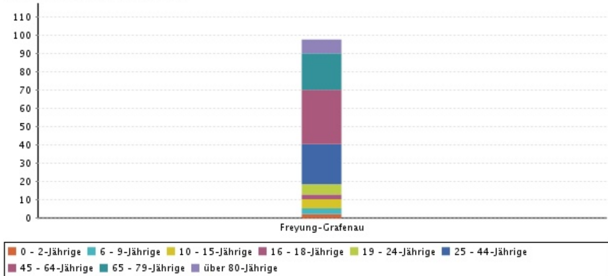
Altersgruppenverteilung 2025 (%)
