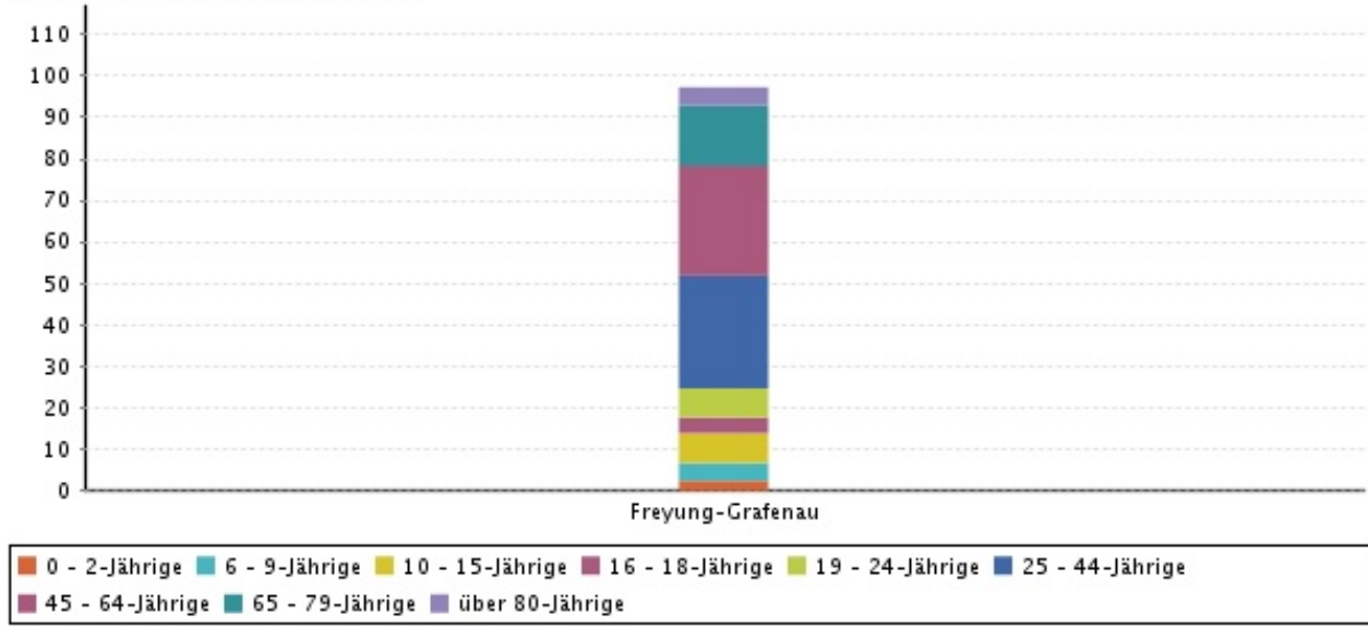
Altersgruppenverteilung 2006 (%)
